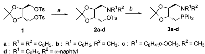
Scheme 1. a: LiNR 1 R 2 , THF, –17 °C; b: LiPPh 2 , THF, 25 °C
